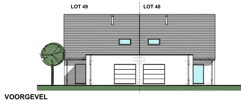
VOORGEVEL
