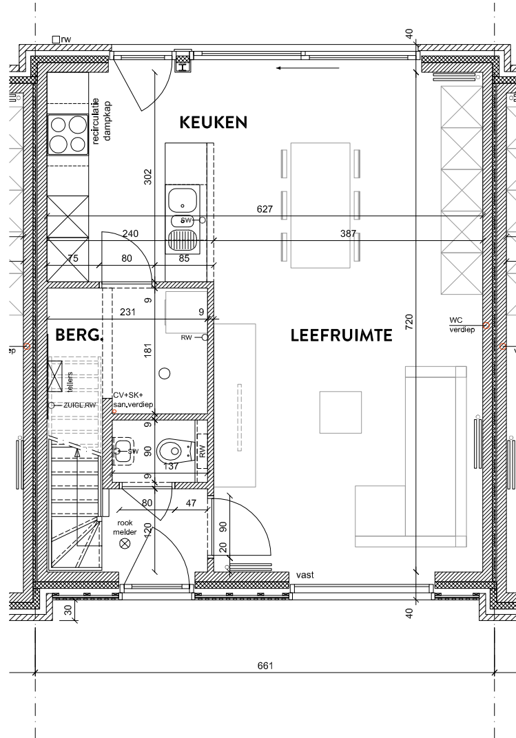
GELIJKVLOERS OPP. 52,4 M 2
