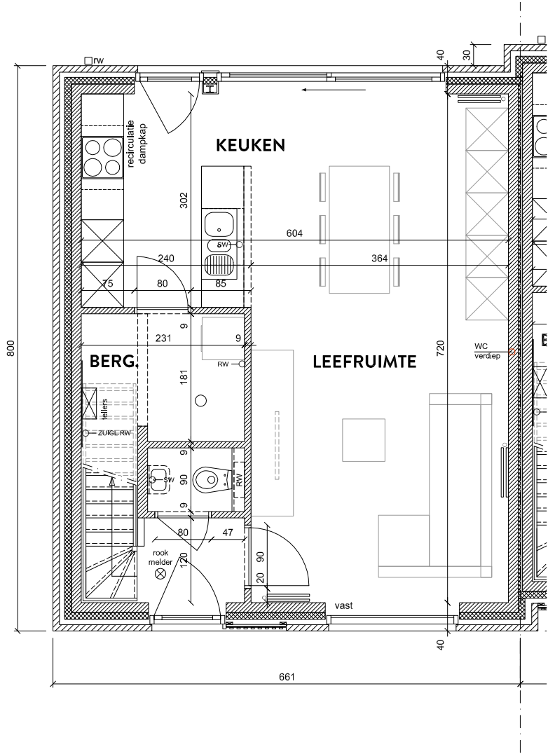
GELIJKVLOERS OPP. 52,64 M 2
