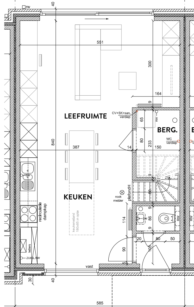
GELIJKVLOERS OPP. 53,27 M 2
