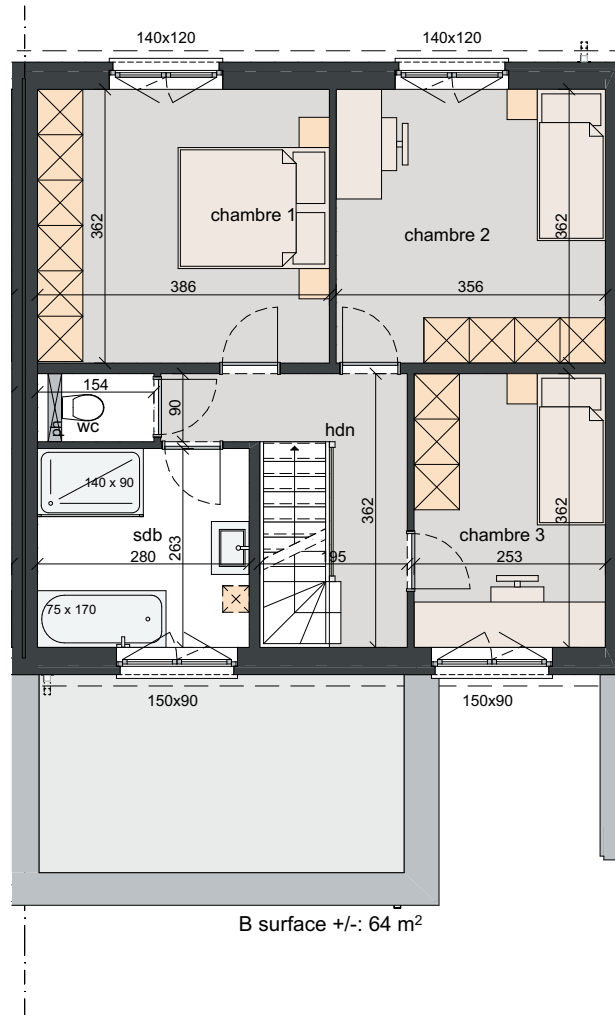
1re étage 1:100
