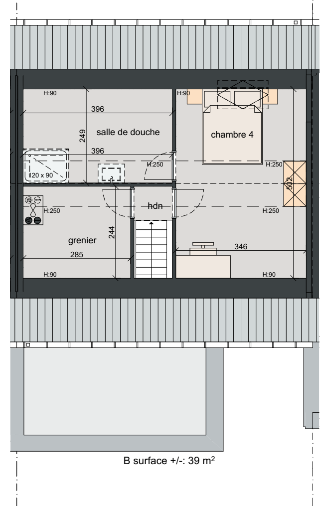
grenier 1:100
