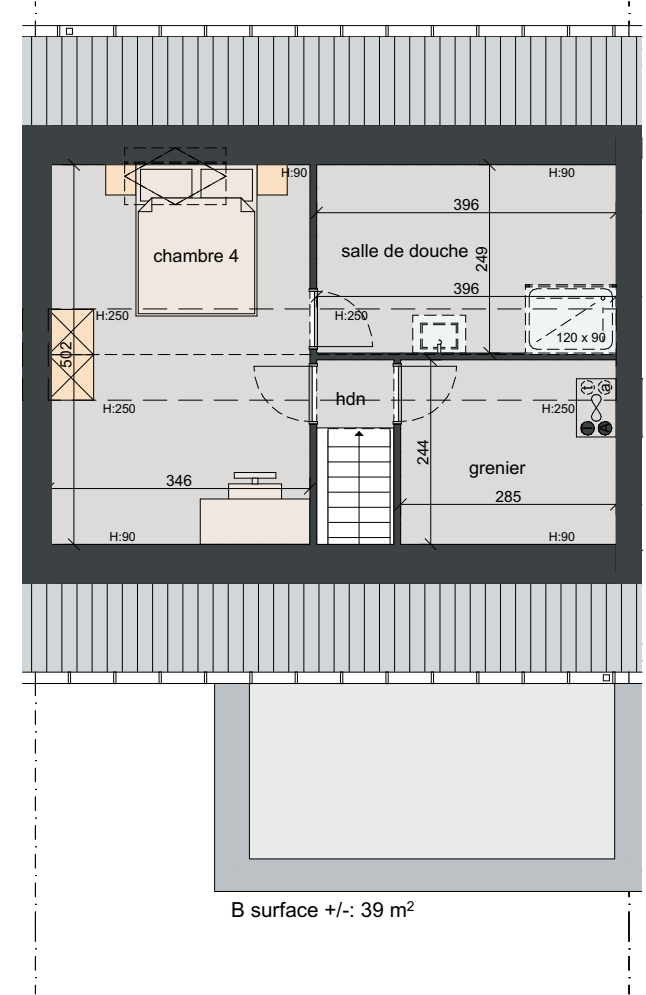
grenier 1:100
