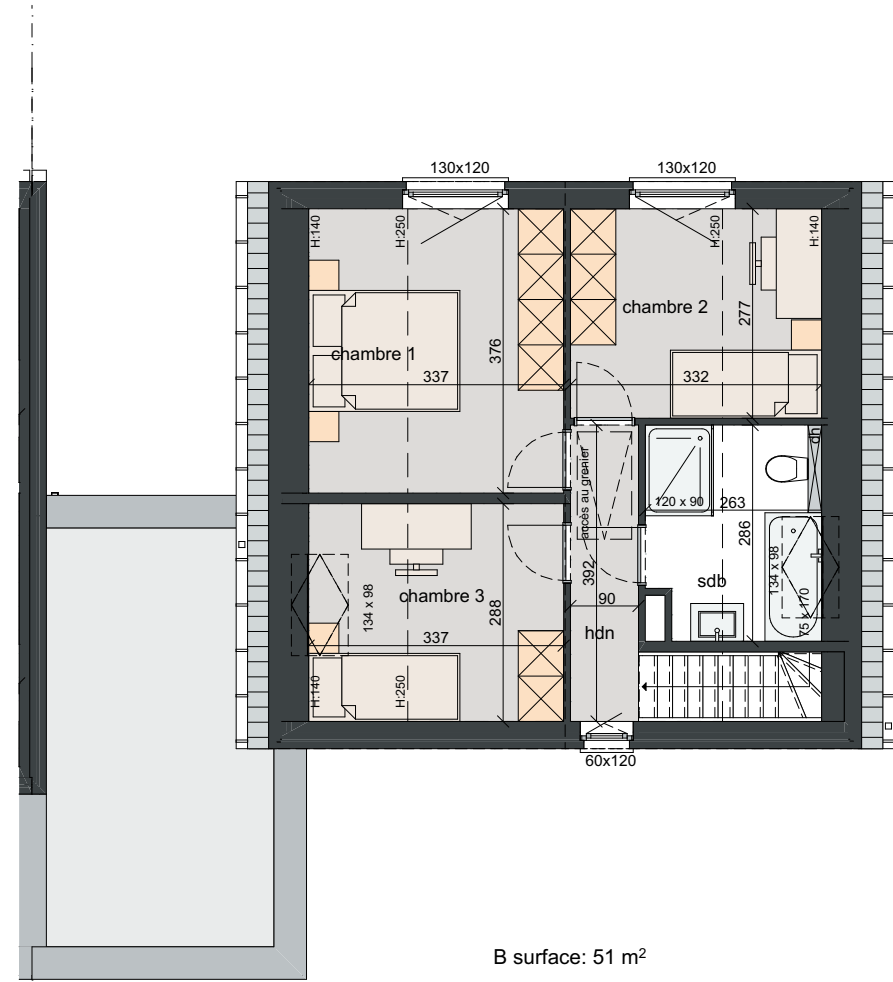
1re étage 1:100
