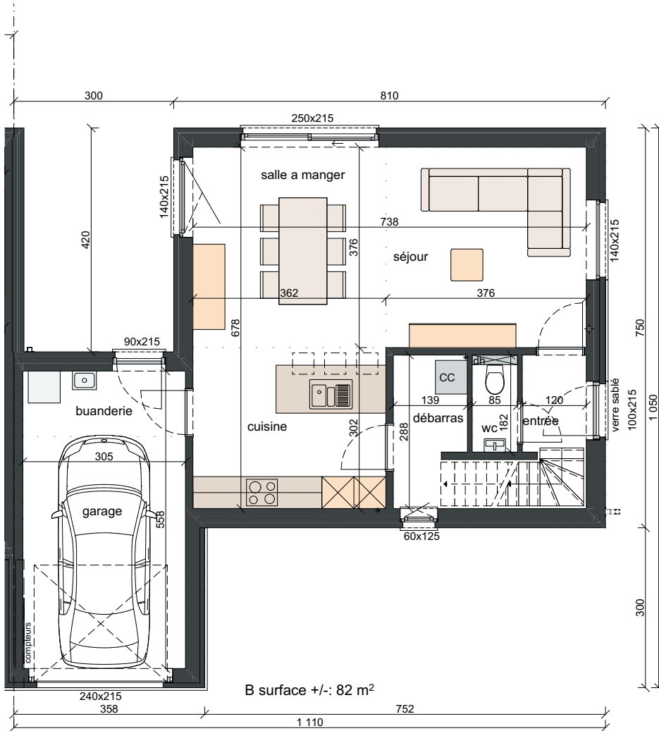
rez-de-chaussée 1:100
