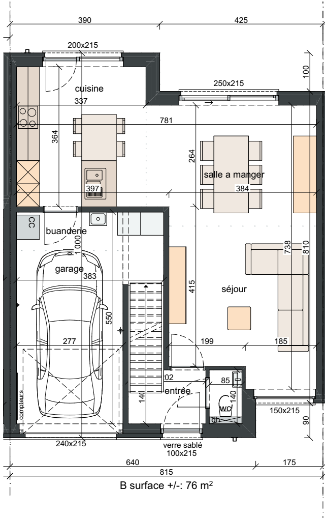
rez-de-chaussée 1:100
