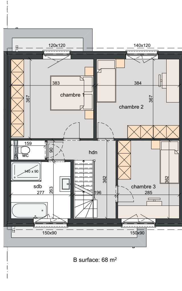
1re étage 1:100
