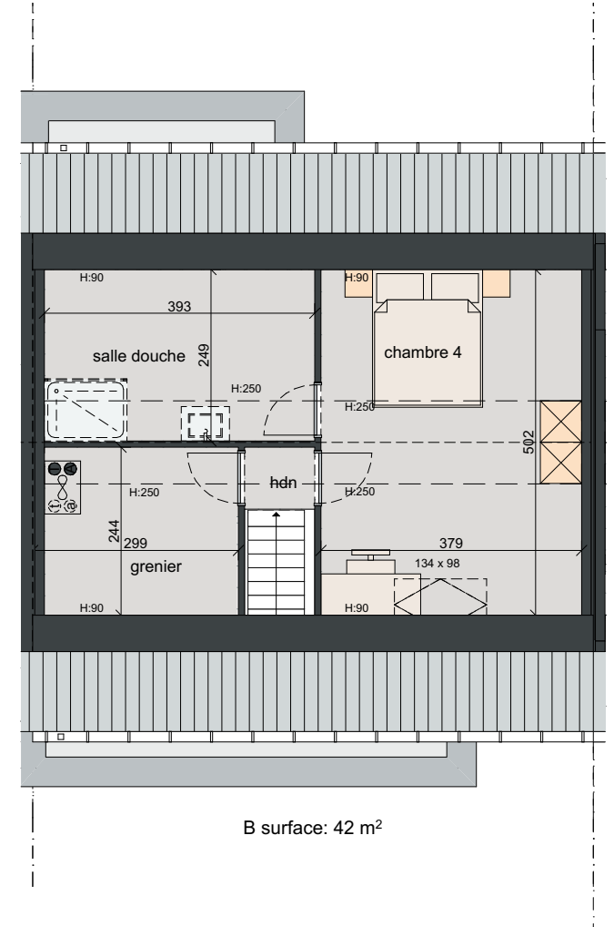
grenier 1:100
