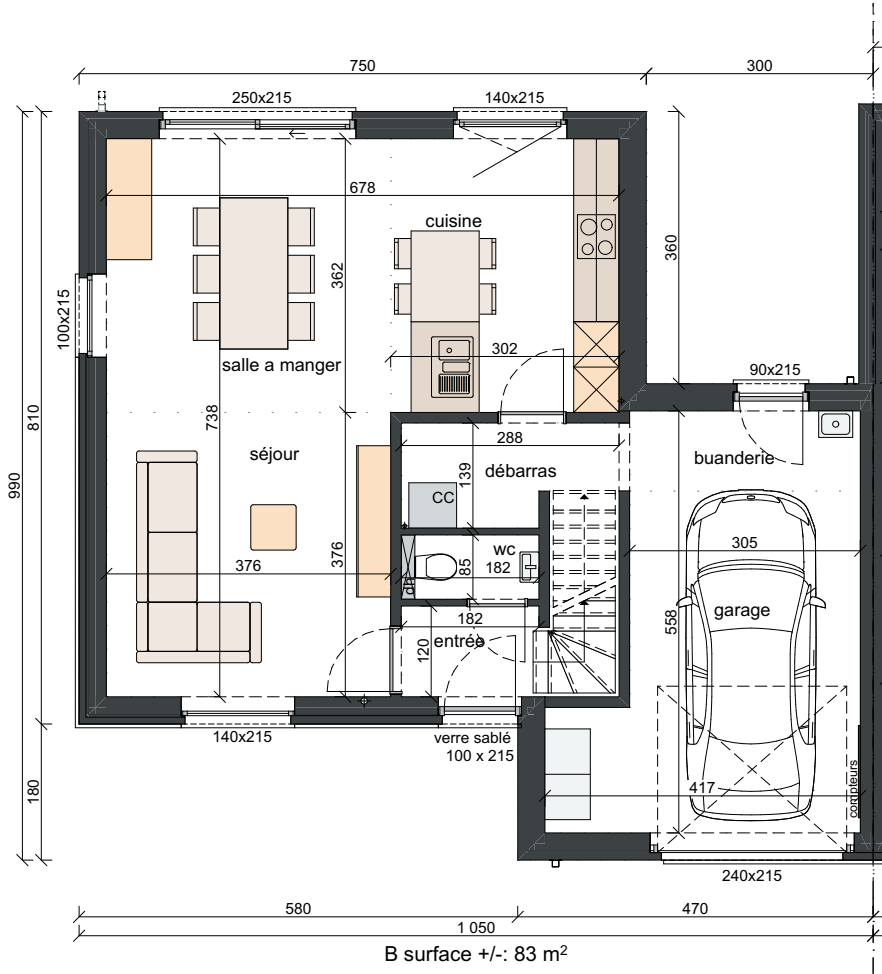
rez-de-chaussée 1:100
