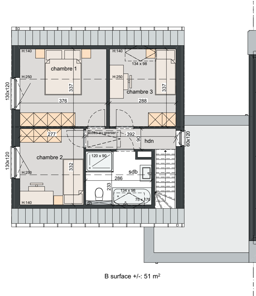
1re étage 1:100
