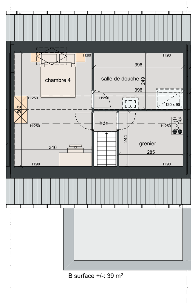
grenier 1:100
