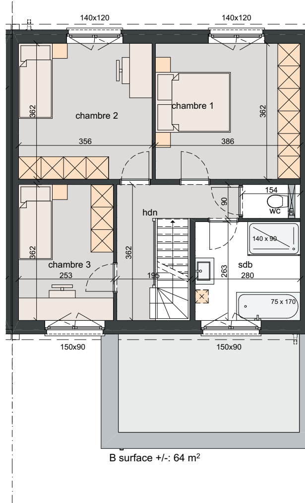
1re étage 1:100
