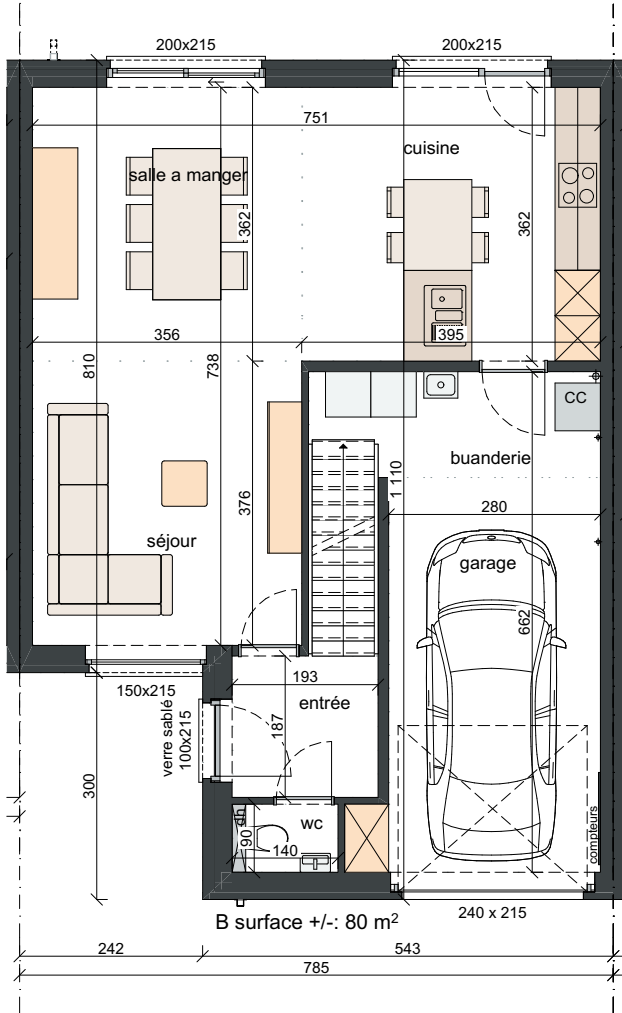
rez-de-chaussée 1:100
