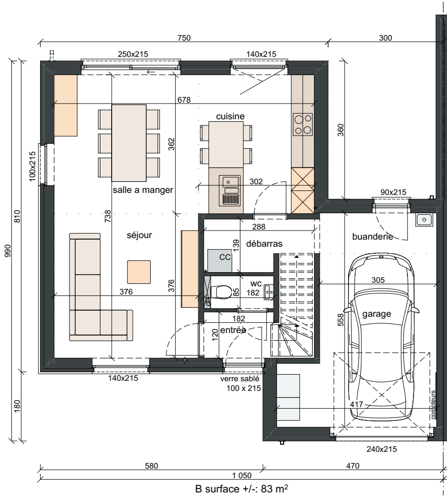
rez-de-chaussée 1:100
