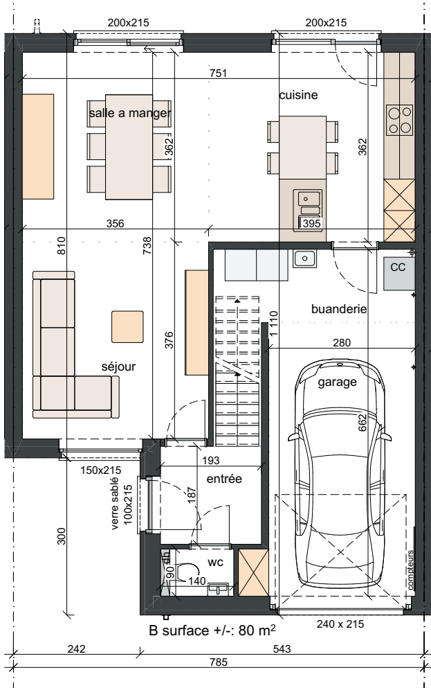
rez-de-chaussée 1:100
