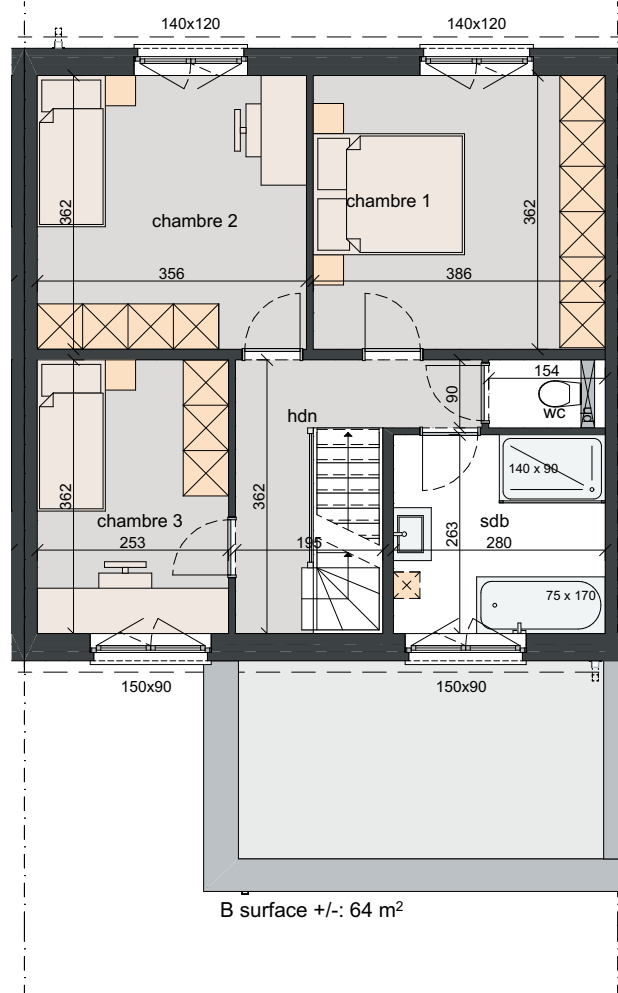
1re étage 1:100
