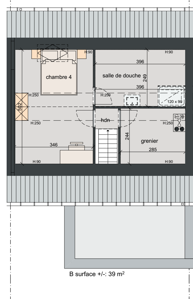
grenier 1:100
