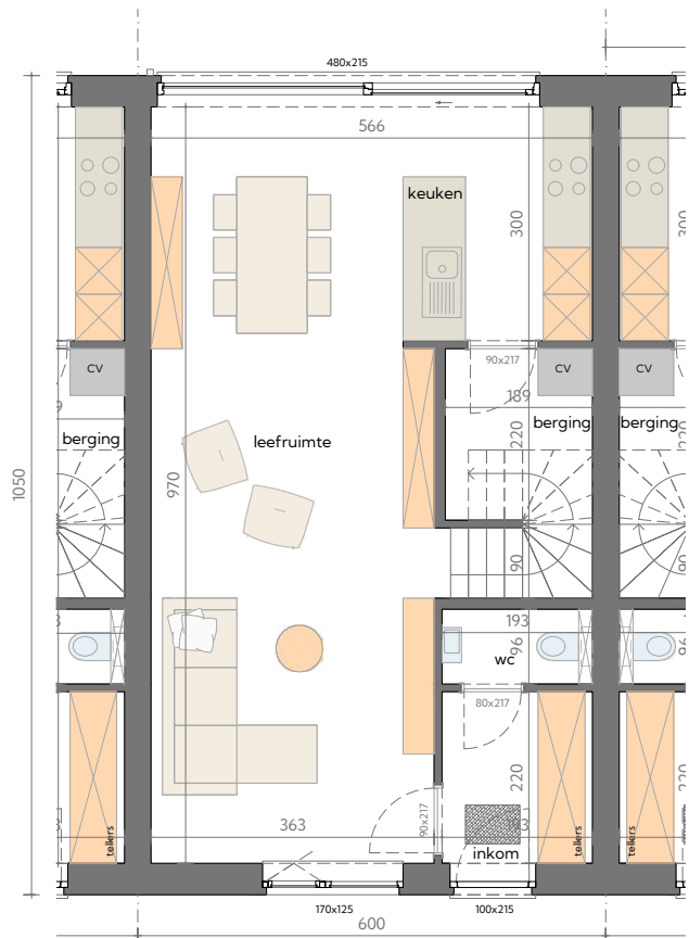
GELIJKVLOERS OPP. 63 M 2
