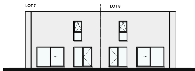
ACHTERGEVEL
