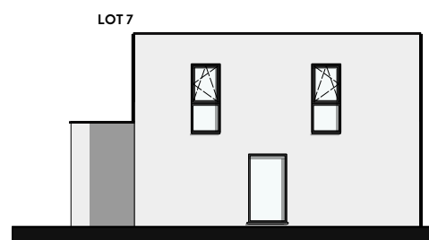
ZIJGEVEL RECHTS
