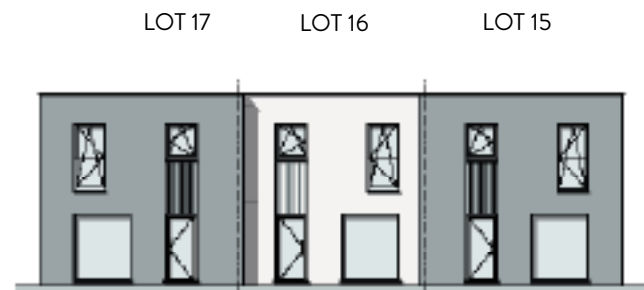
VOORGEVEL
