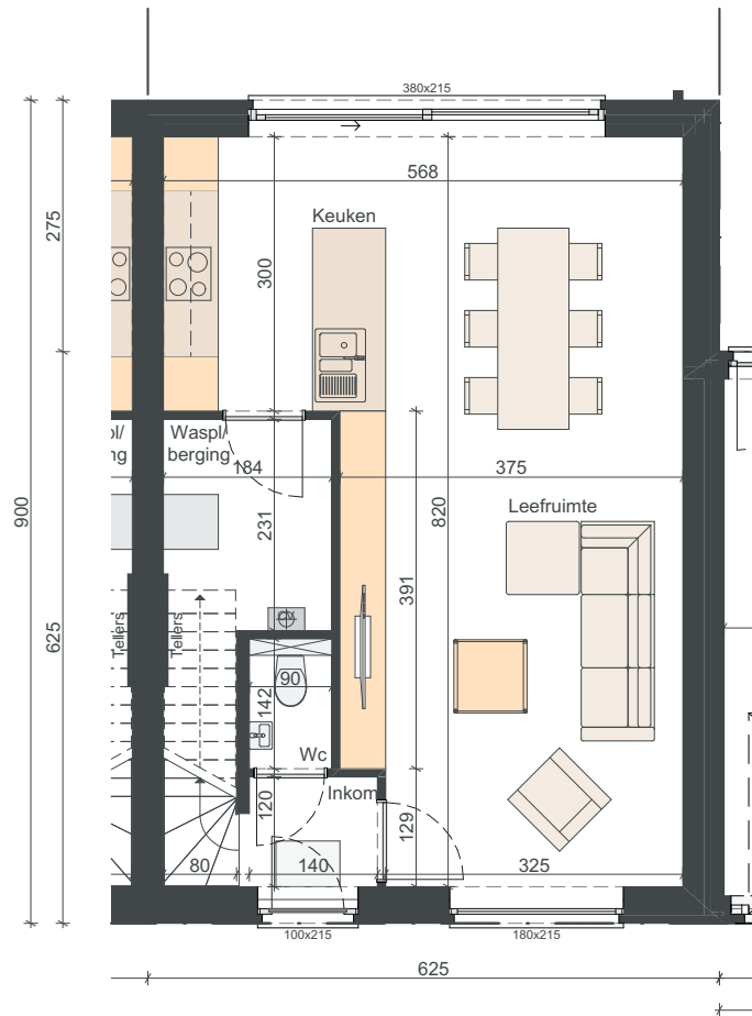
GELIJKVLOERS OPP. ± 56 M 2
