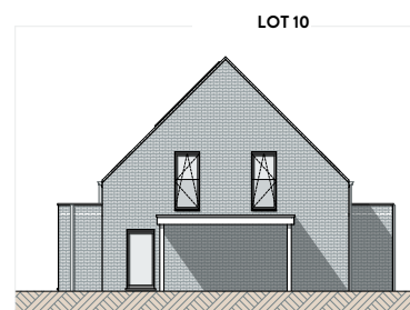
RECHTERGEVEL
