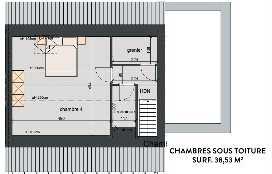
1e étage 1:100
