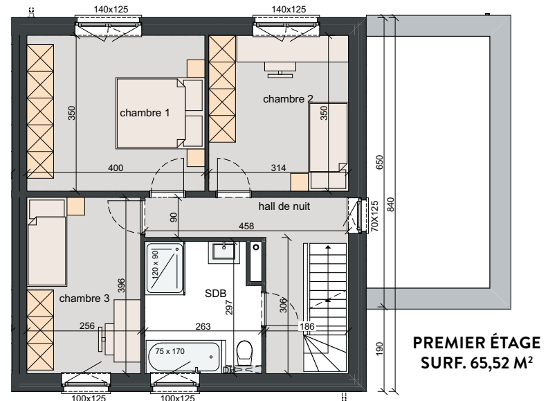
1e étage 1:100
