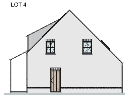
RECHTERGEVEL
