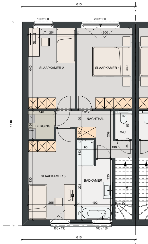
VERDIEPING OPP. = 68,00 m 2
