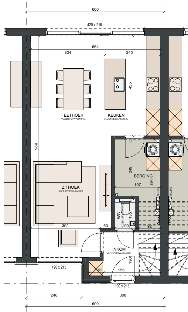
GELIJKVLOERS OPP. = 65,00 m 2
