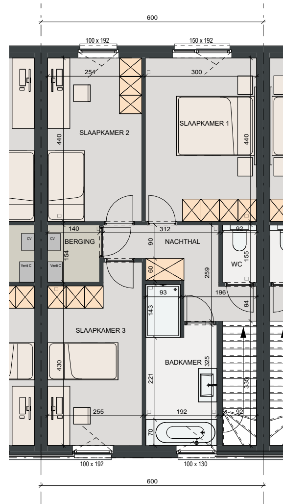
VERDIEPING OPP. = 67,00 m 2
