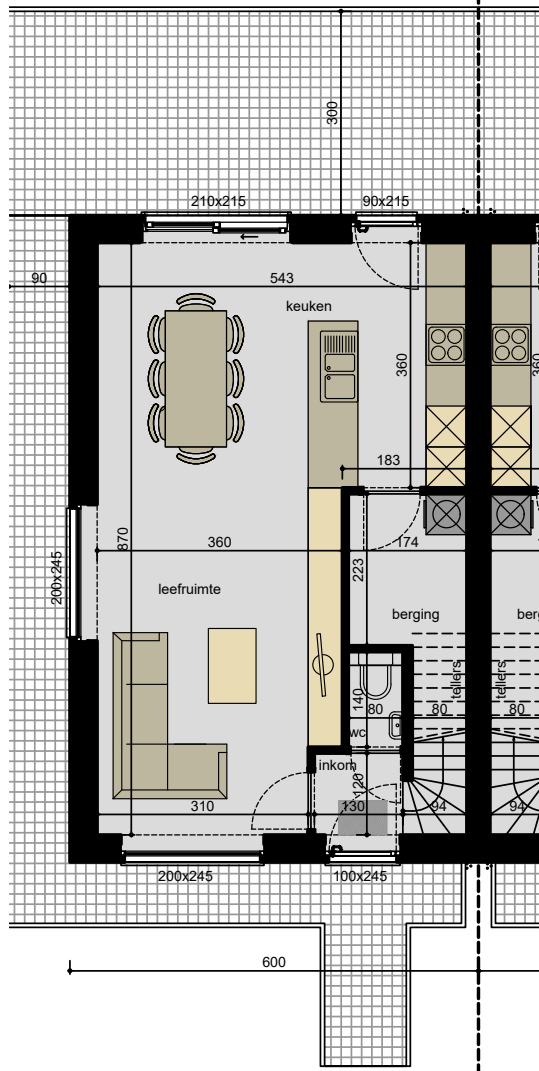
GELIJKVLOERS OPP. 57,00M 2
