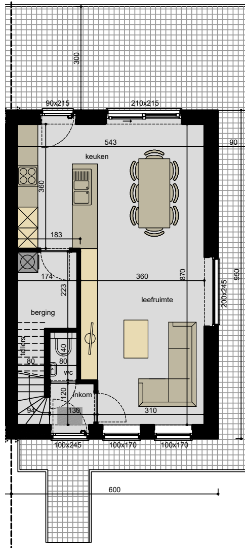
GELIJKVLOERS OPP. 57,00M 2
