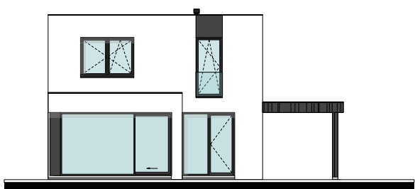
ACHTERGEVEL
