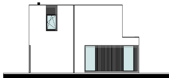
RECHTERGEVEL
