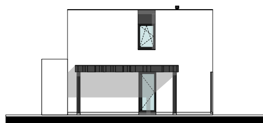
LINKERGEVEL
