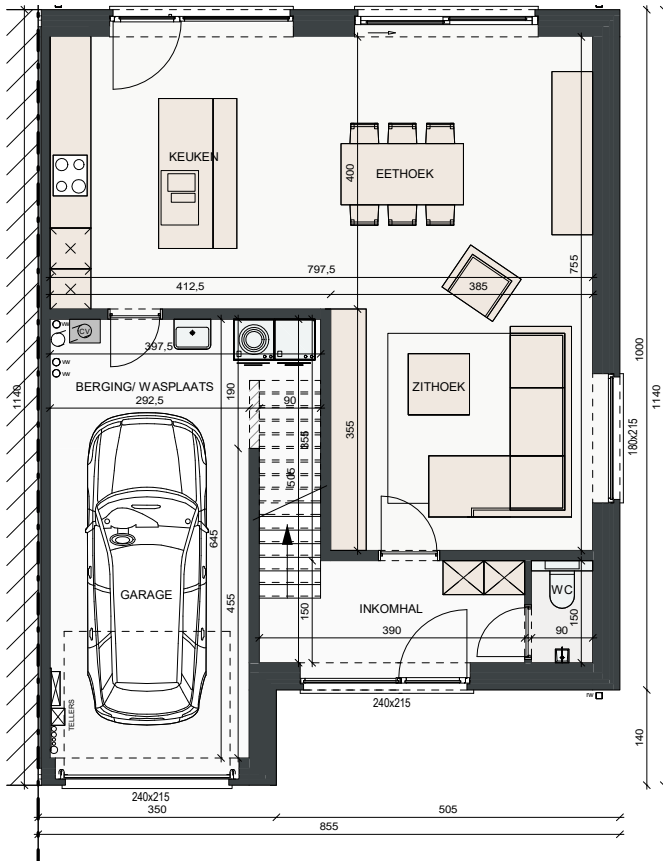
GELIJKVLOERS OPP. 90,40 M 2
