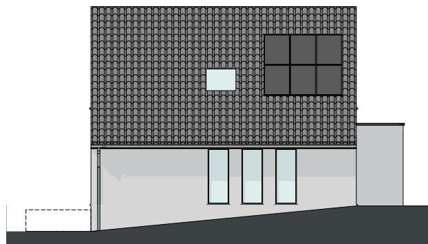
ZIJGEVEL LINKS
