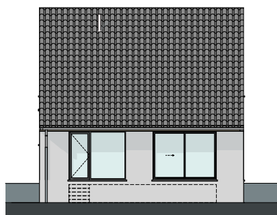
ACHTERGEVEL
