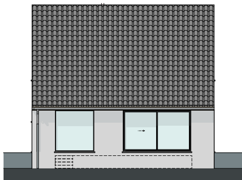
ACHTERGEVEL
