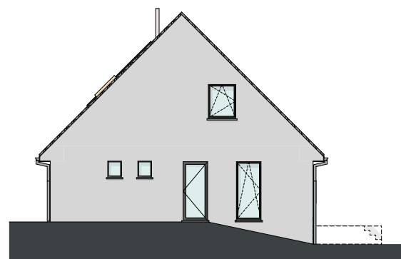
ZIJGEVEL RECHTS
