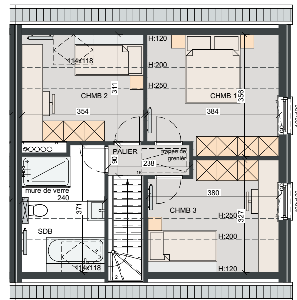
PREMIÈRE ÉTAGE SURF. 65,60 M 2
