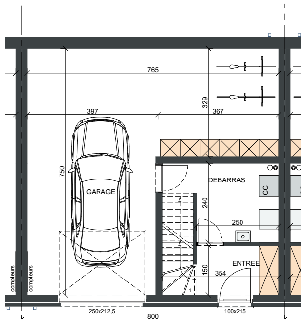
SOUS-SOL SURF. 65,60 M 2
