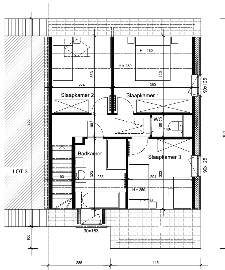
VERDIEPING OPP. = 56,50 m 2
