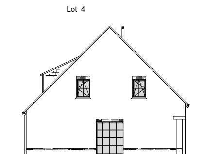
ZIJGEVEL
