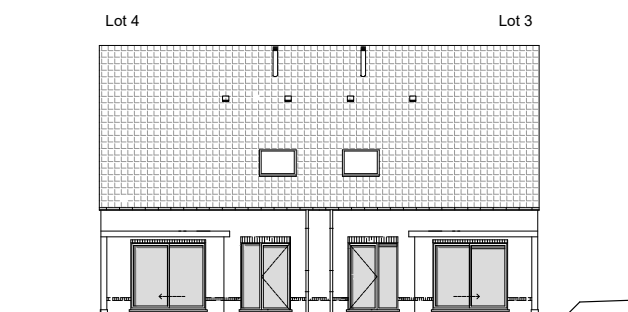
ACHTERGEVEL
