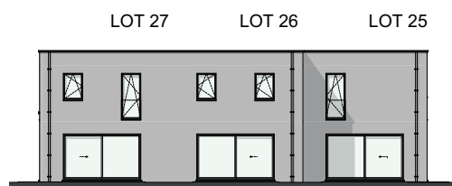
RECHTERGEVEL
