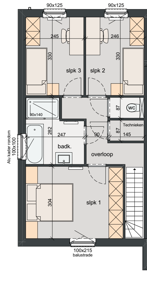
VERDIEPING OPP 54,89 M 2
