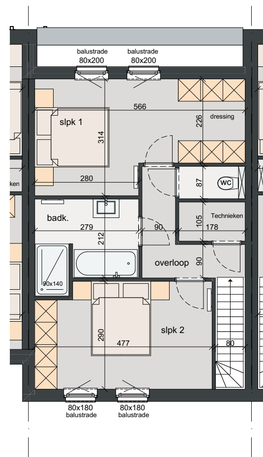
VERDIEPING OPP. 53,74 M 2
