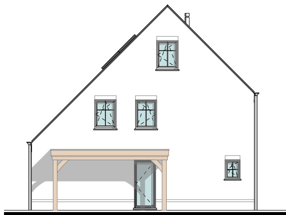
ZIJGEVEL LINKS
