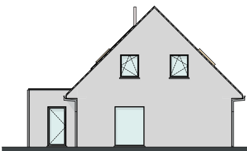
ZIJGEVEL RECHTS
