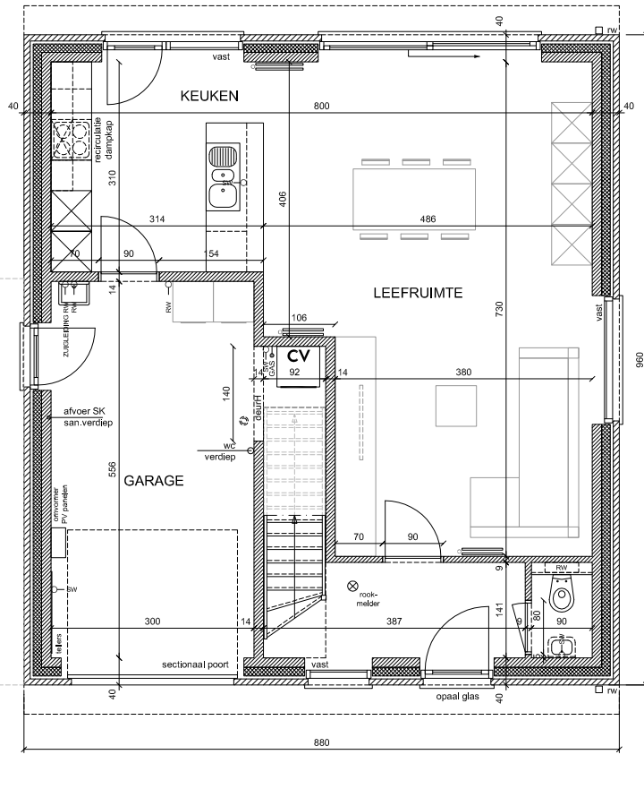
GELIJKVLOERS OPP. 84,48 M 2
