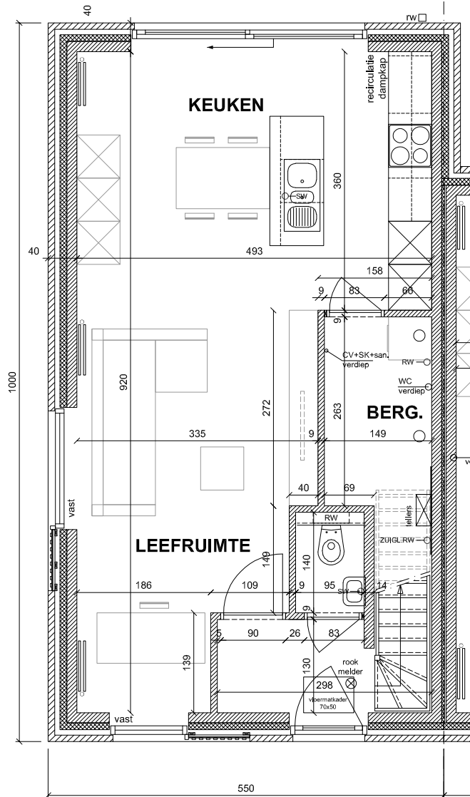
GELIJKVLOERS OPP. 54,7 M 2
