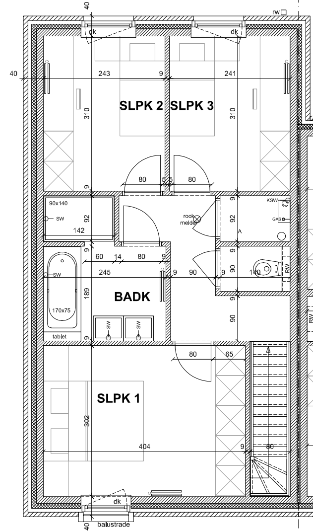
VERDIEPING OPP. 54,7 M 2
