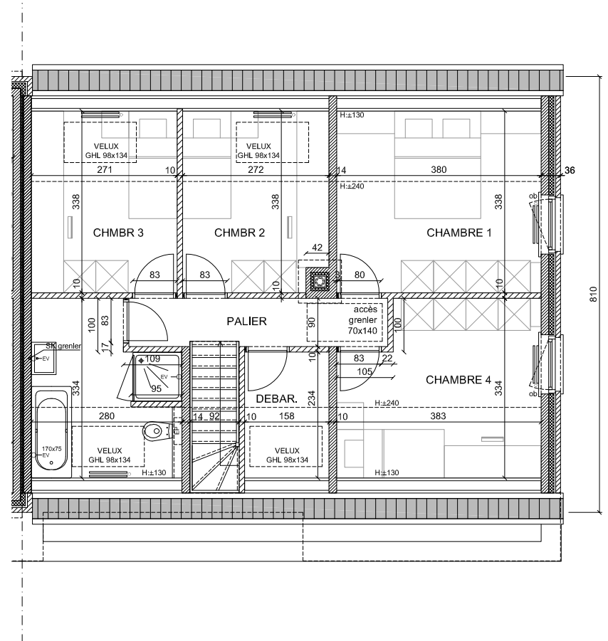
ÉTAGE SURF. 68,00 M 2
