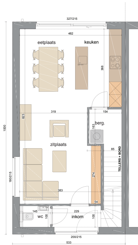
GELIJKVLOERS OPP. 53M 2
