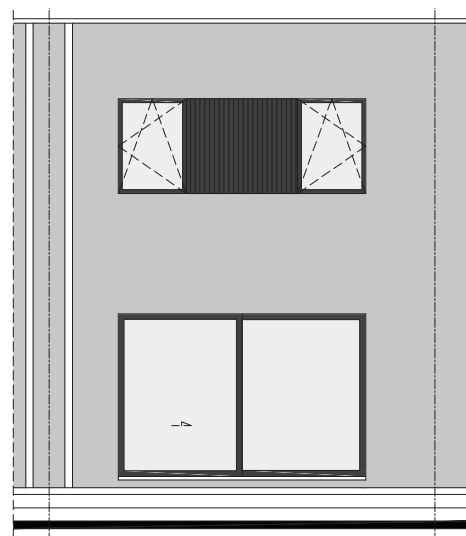
ACHTERGEVEL
