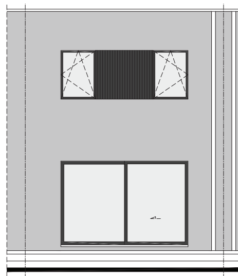
ACHTERGEVEL
