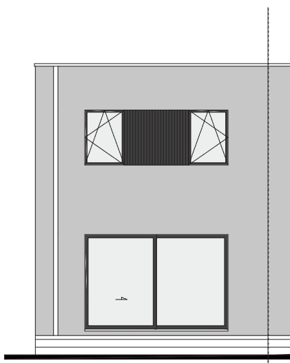
ACHTERGEVEL
