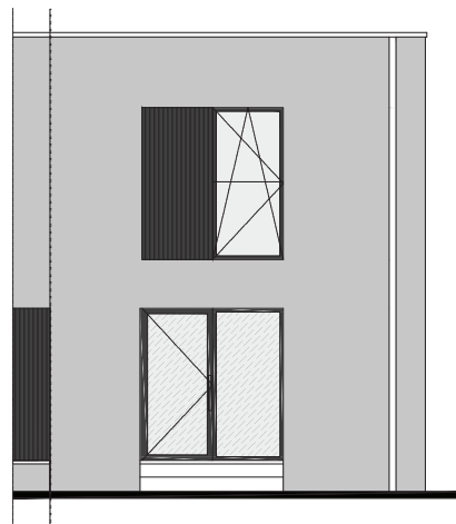
VOORGEVEL
