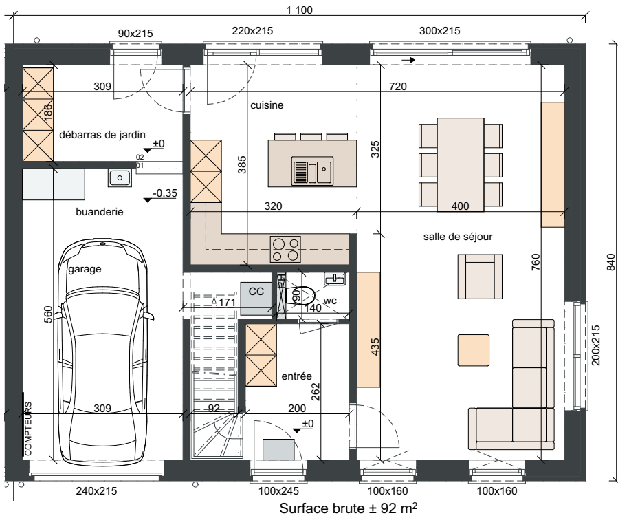
rez de chaussée 1:100
