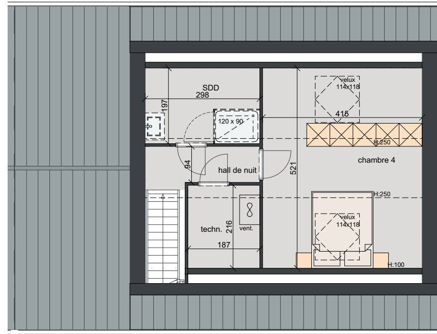
2e étage 1:100
