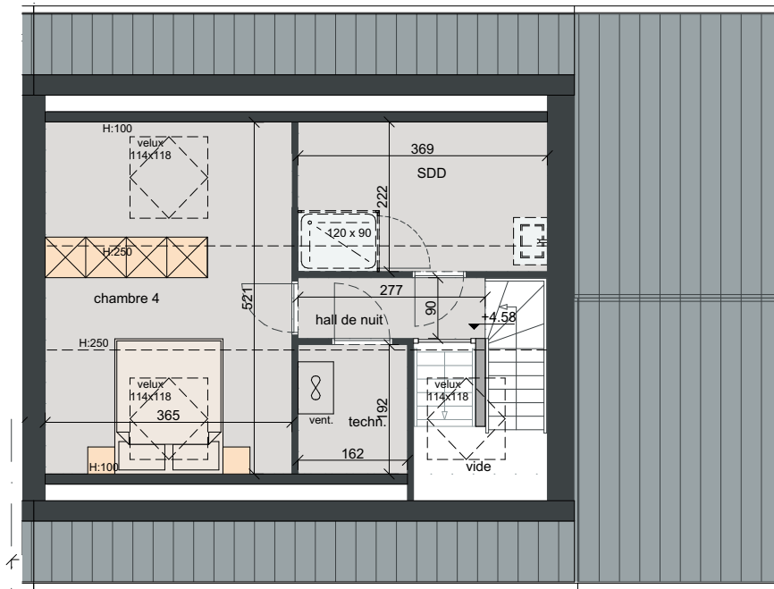
2e étage 1:100 Surface brute ± 43 m 2
