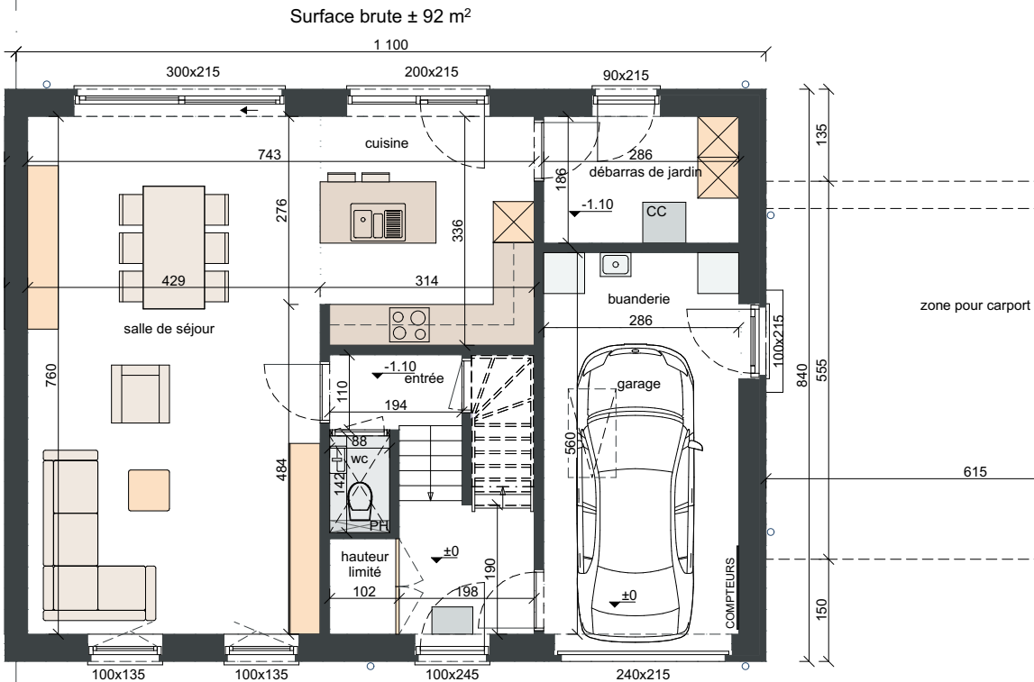
rez de chaussée 1:100
