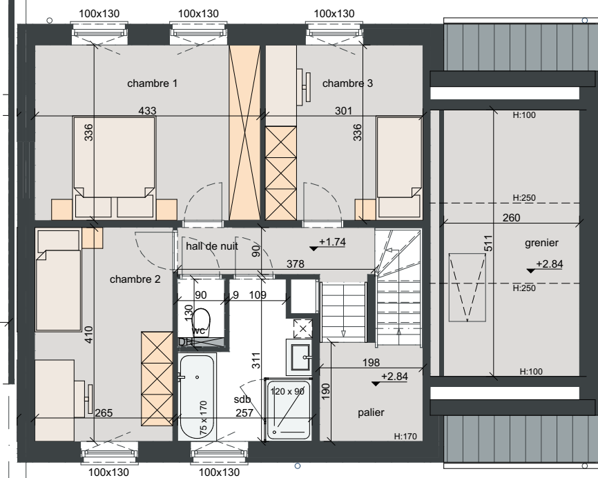
1e étage 1:100 Surface brute ± 81 m 2
