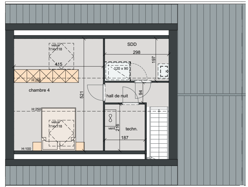
2e étage 1:100 Surface brute ± 42 m 2
