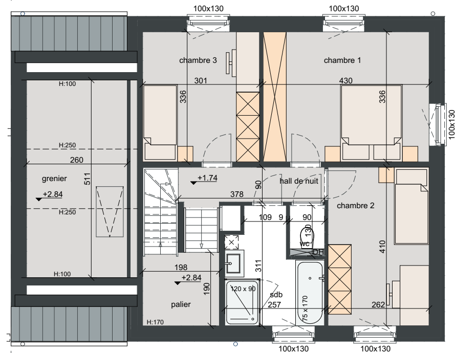
1e étage 1:100
