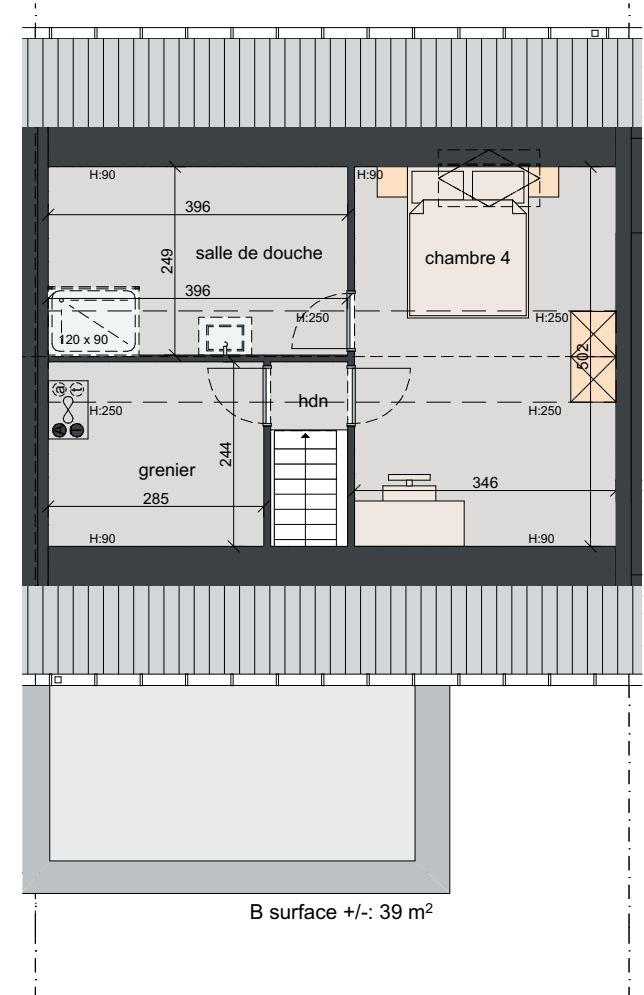
grenier 1:100
