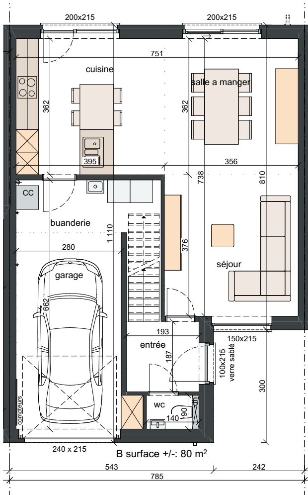
rez-de-chaussée 1:100
